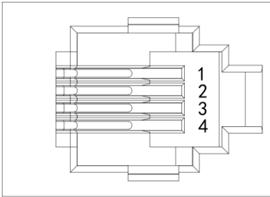
(3) RJ11 计量检测接口管脚定义示意图
