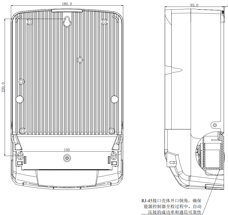
图 4 终端侧视/后视尺寸示意图
